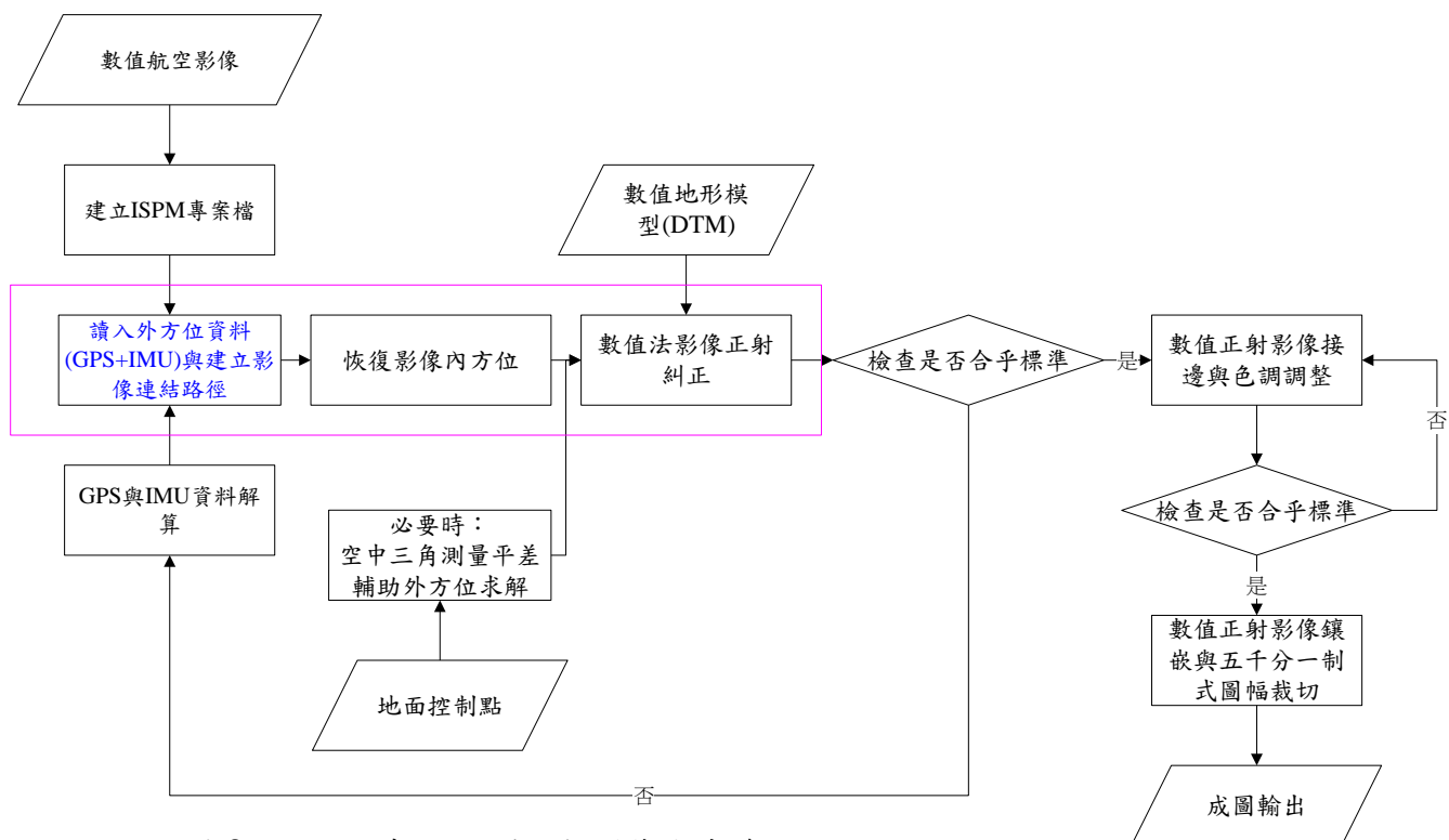
圖 3、現階段數值航測正射影像生產流程
