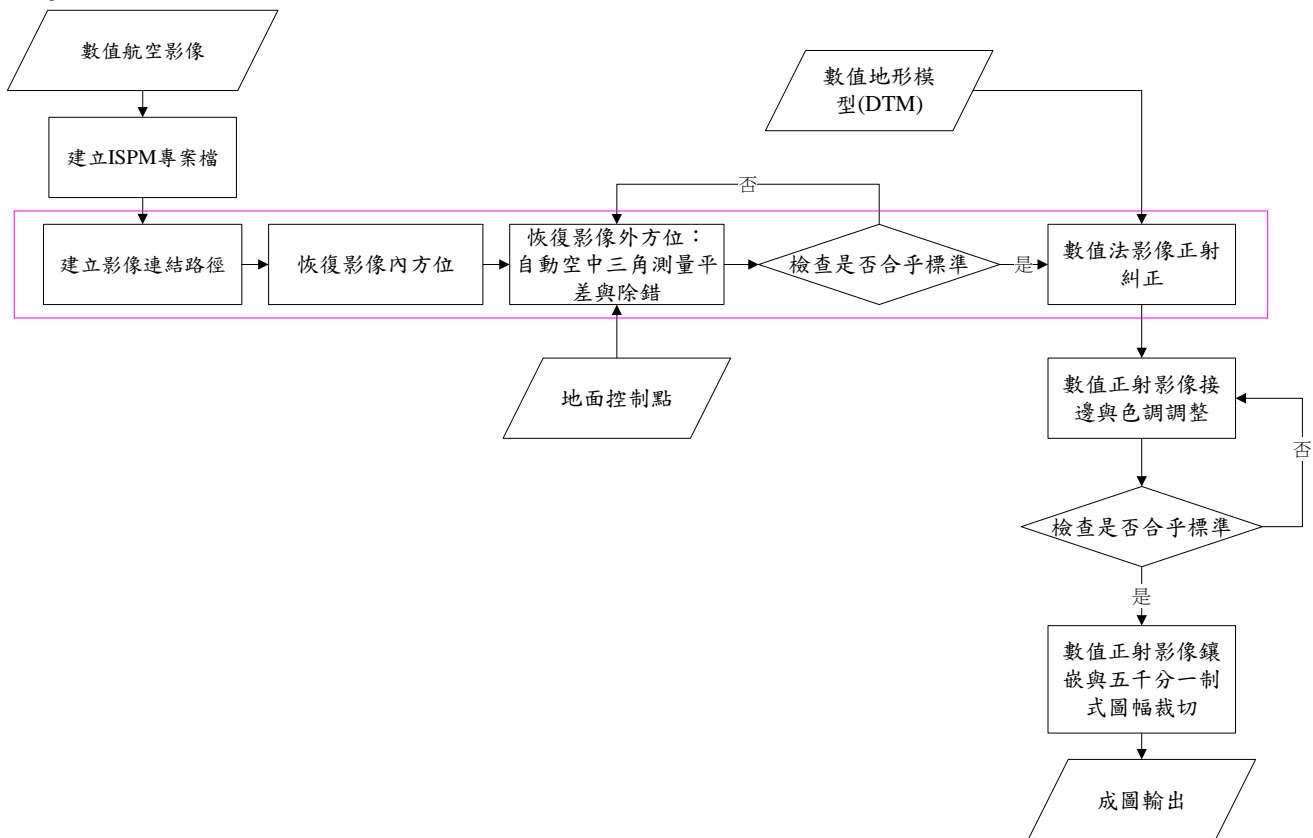
圖 2、過去數值航測正射影像生產流程
